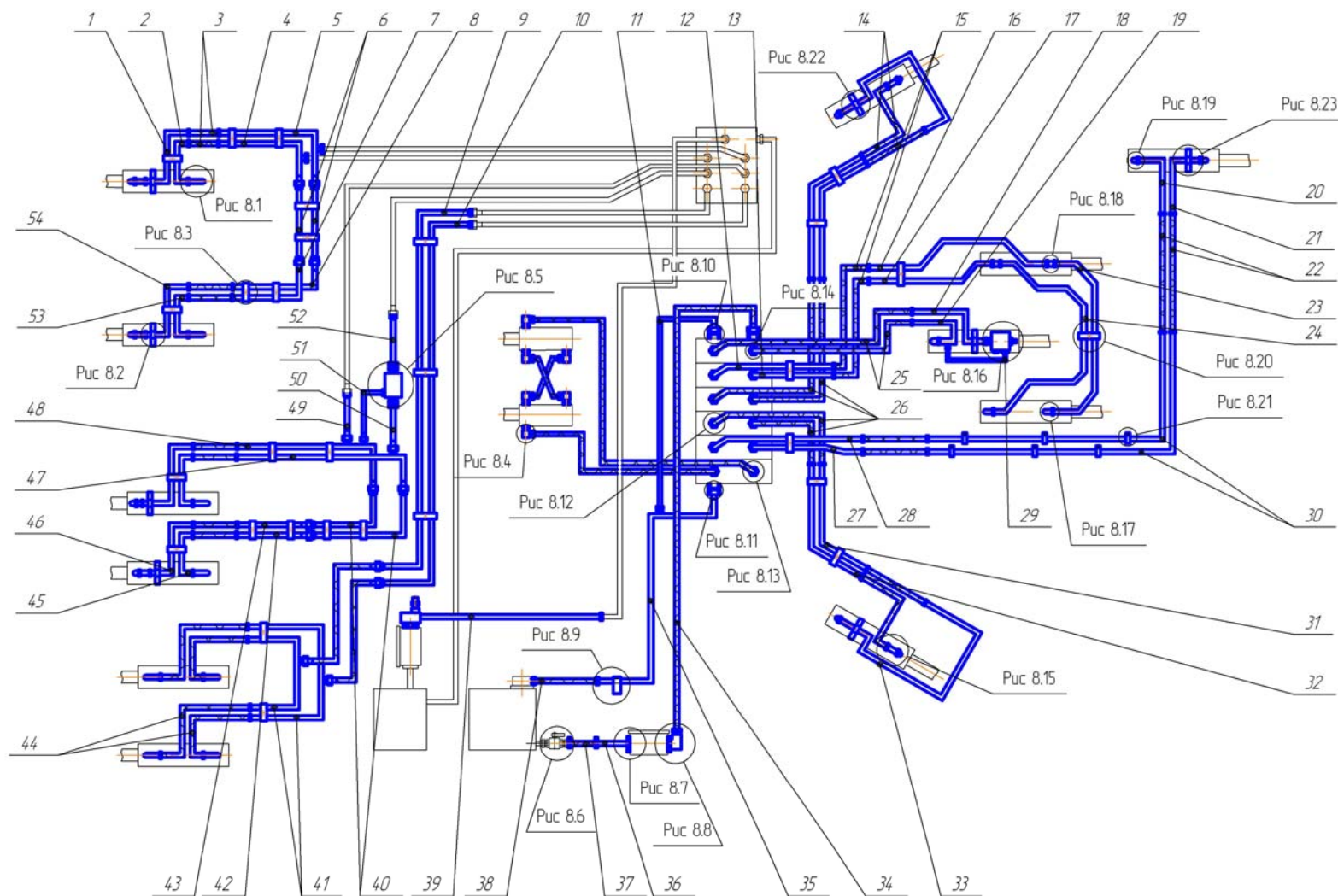
Рис. 8 Гидроразводка
