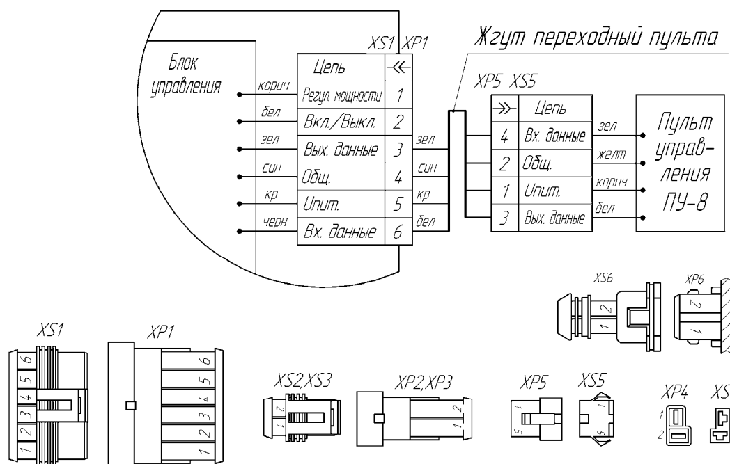
Схема подключения пульта ПУ-8**
