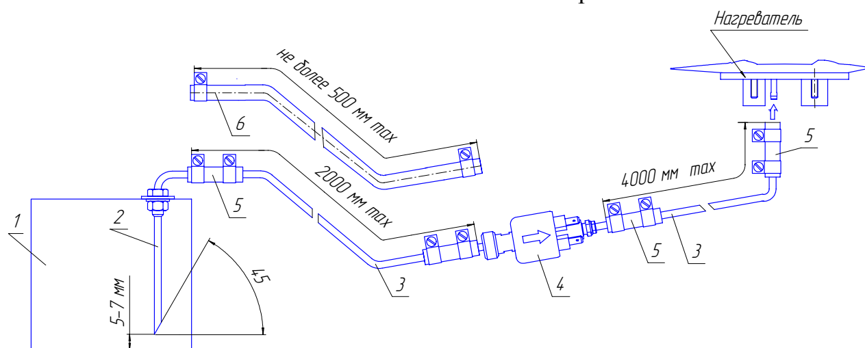
Рис. 8.4 – Монтаж топливозаборника.
