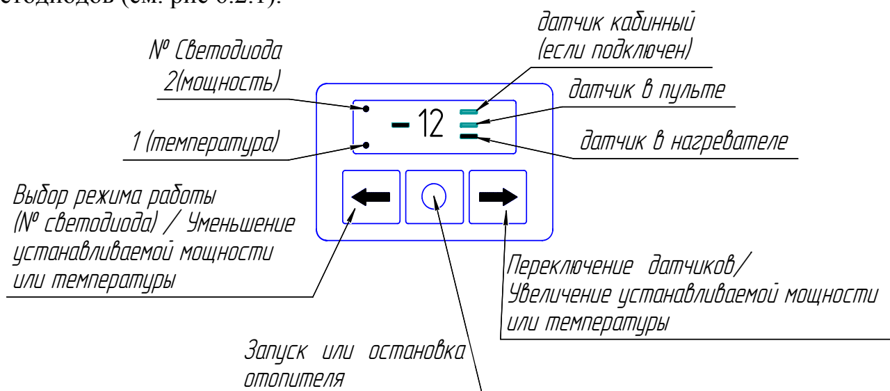
Рис. 6.2.1- Панель пульта
