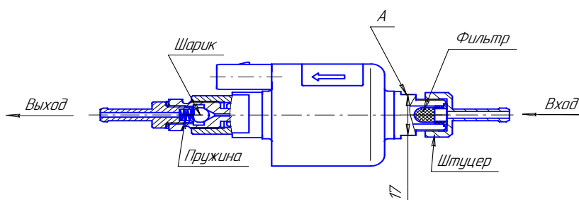
Рис.10.1 – Топливный насос
