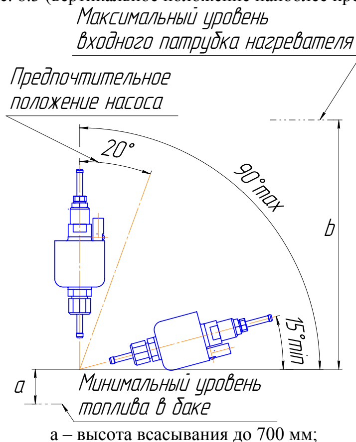
Рис. 8.3 - Допустимое монтажное положение топливного насоса.
